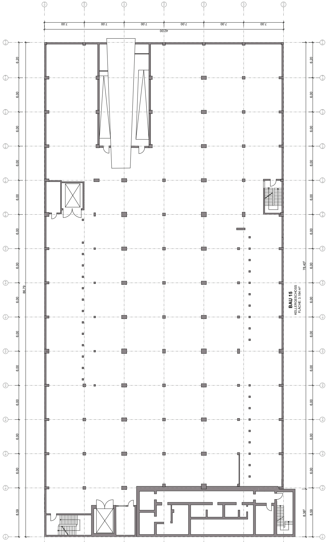
Bau 15 Grundriss Kellergeschoss
