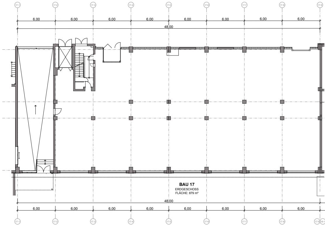
Bau 17 Grundriss Erdgeschoss
