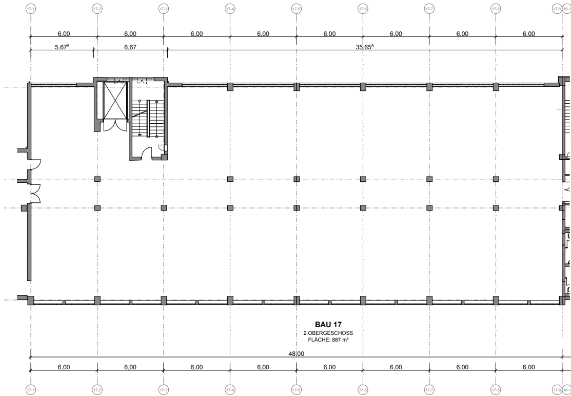
Bau 17 Grundriss 2.Obergeschoss
