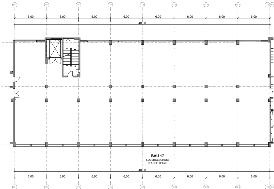
Bau 17 Grundriss 1.Obergeschoss
