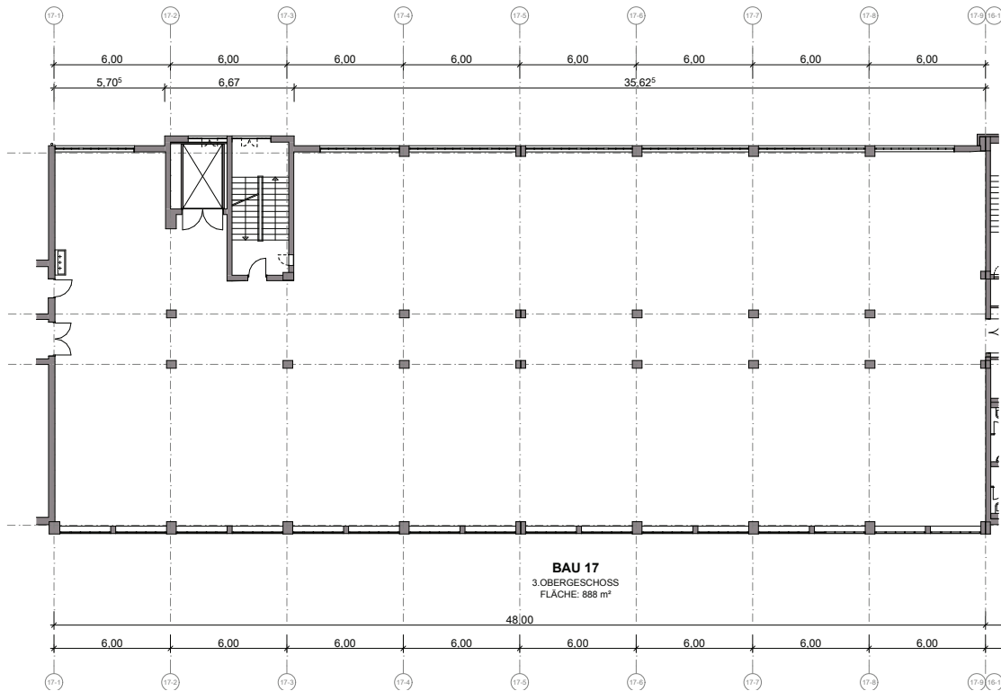
Bau 17 Grundriss 3.Obergeschoss
