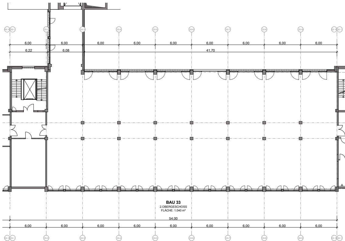
Bau 33 Grundriss 2.Obergeschoss
