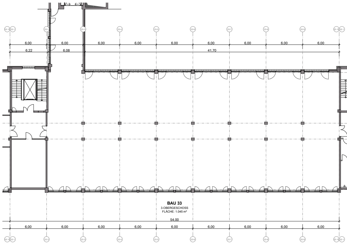
Bau 33 Grundriss 3.Obergeschoss
