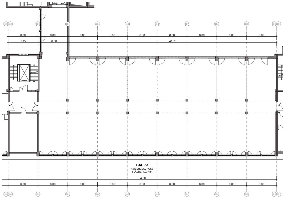
Bau 33 Grundriss 1.Obergeschoss
